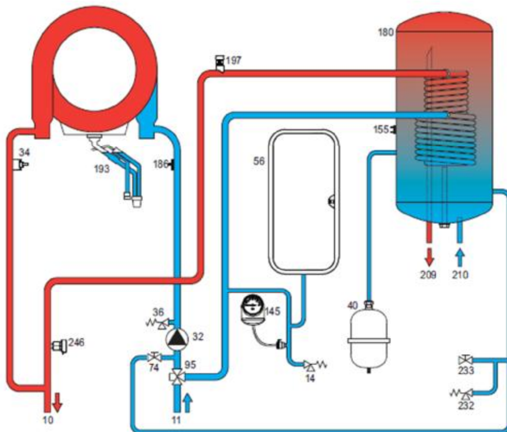
48. ábra – hidraulikai séma
