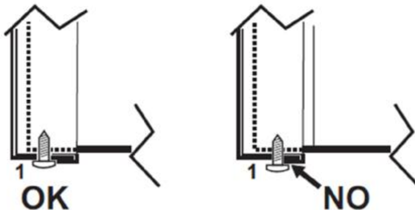
ábra. 42- Előlap korrekt pozíciója
